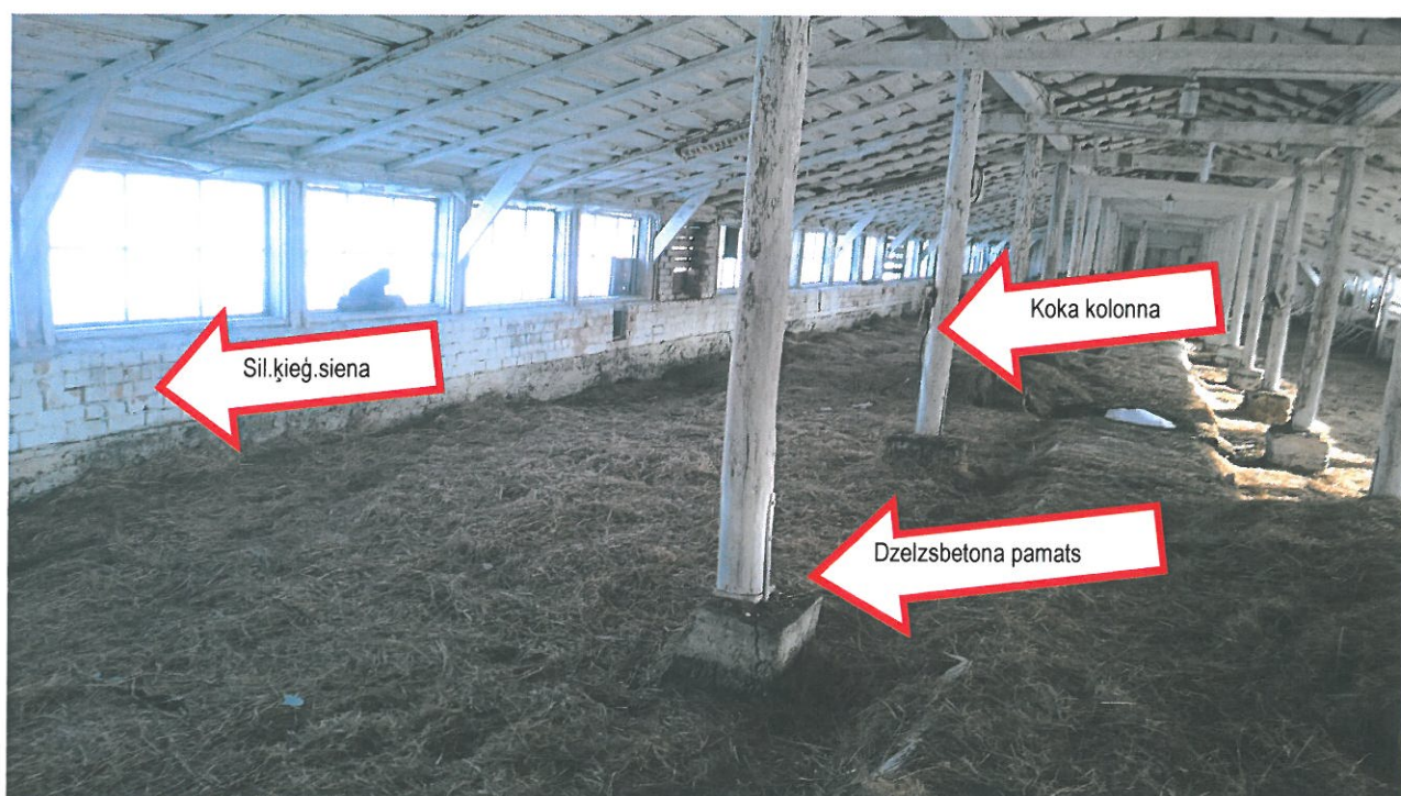
5.attēls. Demontējamas ēkas konstrukcijas.
